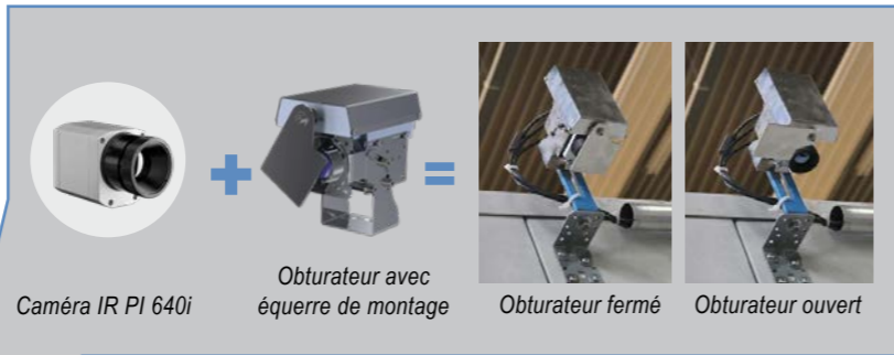
Surveillance des températures de feuilles de verre dans une installation de trempage
