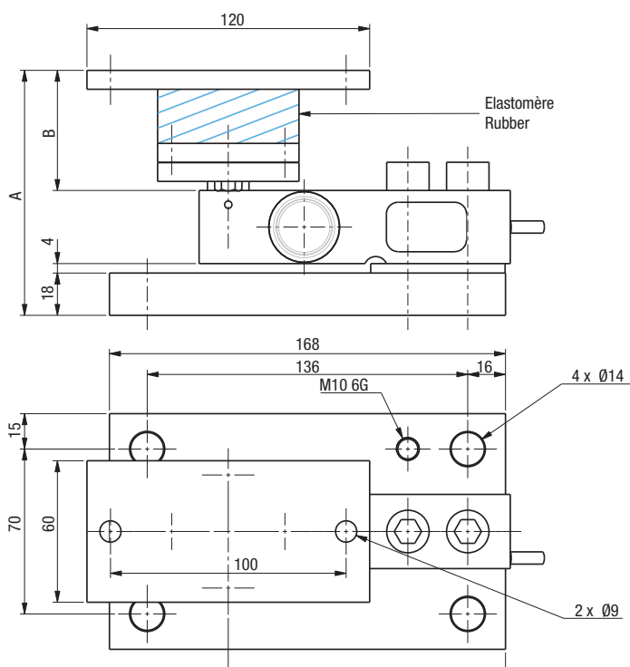
Encombrement et fixation - Dimensions and fixing
