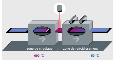
Caméra infrarouge avec fonction caméra linéaire
