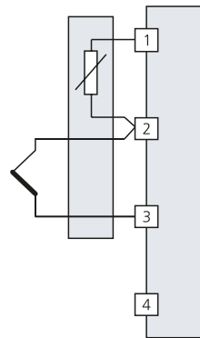
Thermocouple avec compensation externe des jonctions de référence
