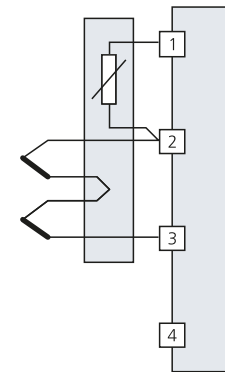
Thermocouples en circuit de connexion additionneur (détermination de la moyenne), compensation externe des jonctions de référence
